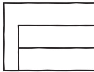
Wiederholung/Schleife
