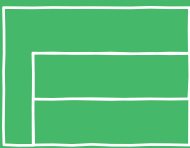
Schleifen
