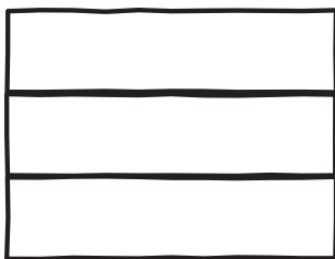
Anweisung
