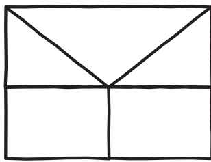
Entscheidung/Abfrage
