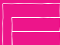
Schleifen
