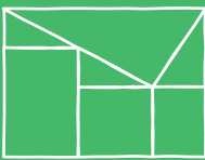
Abfragen (mehrfach)
